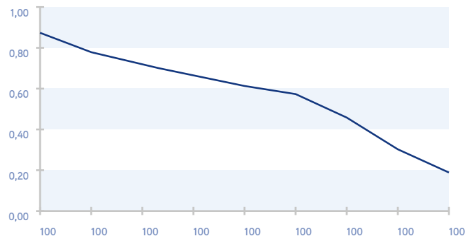
Gráfico 1: Factor de reducción de temperatura para la presión de trabajo:
